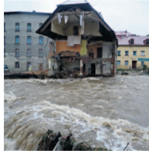
Zřícený dům v Chrastavě
